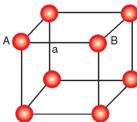
Fig. 23 Simple cubic.
