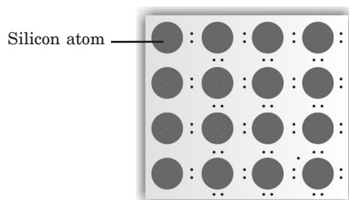
Fig. 1. Pure crystal
